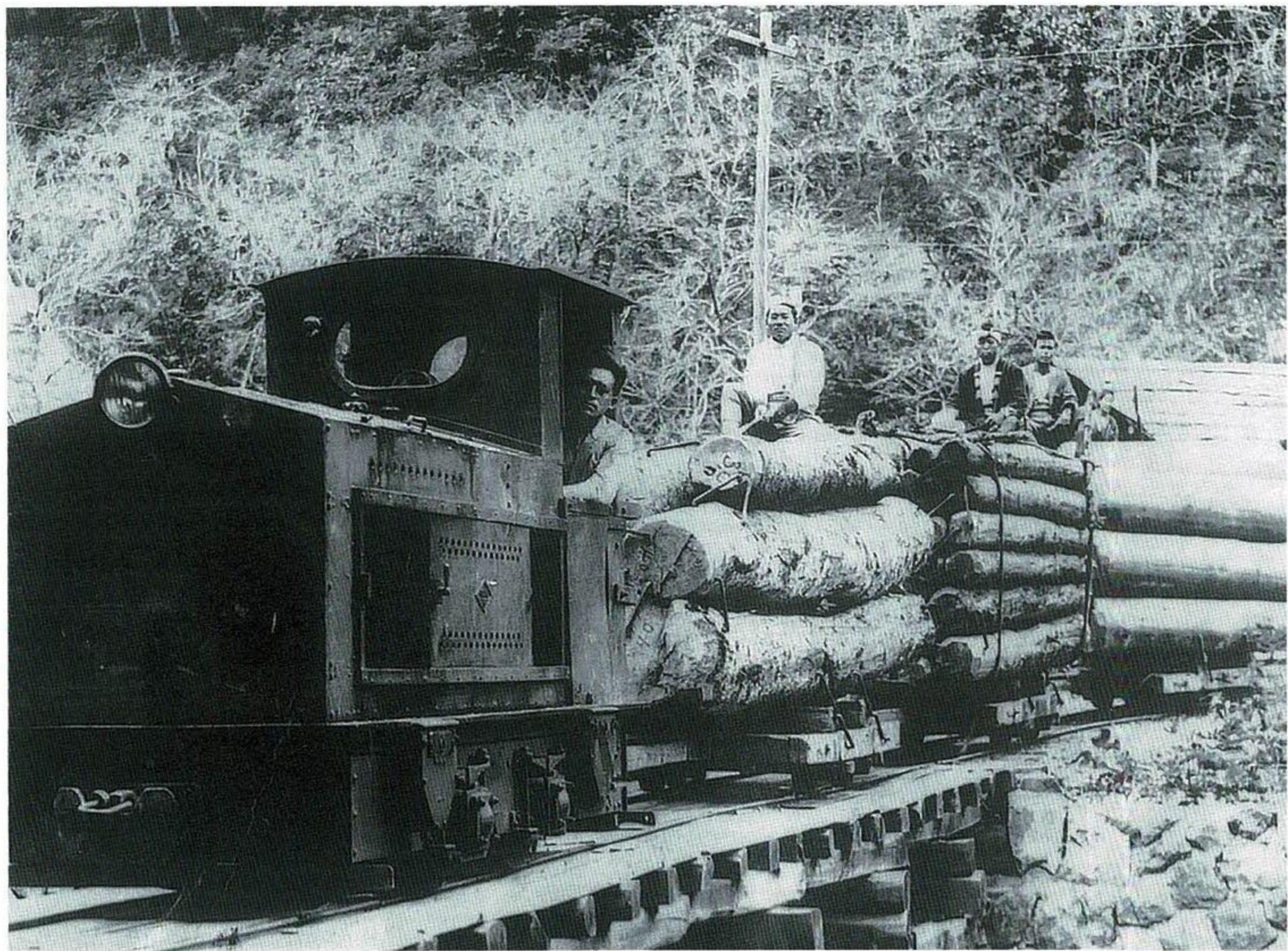
赤西国有林事務所下の森林鉄道（橋元利之氏 提供）
