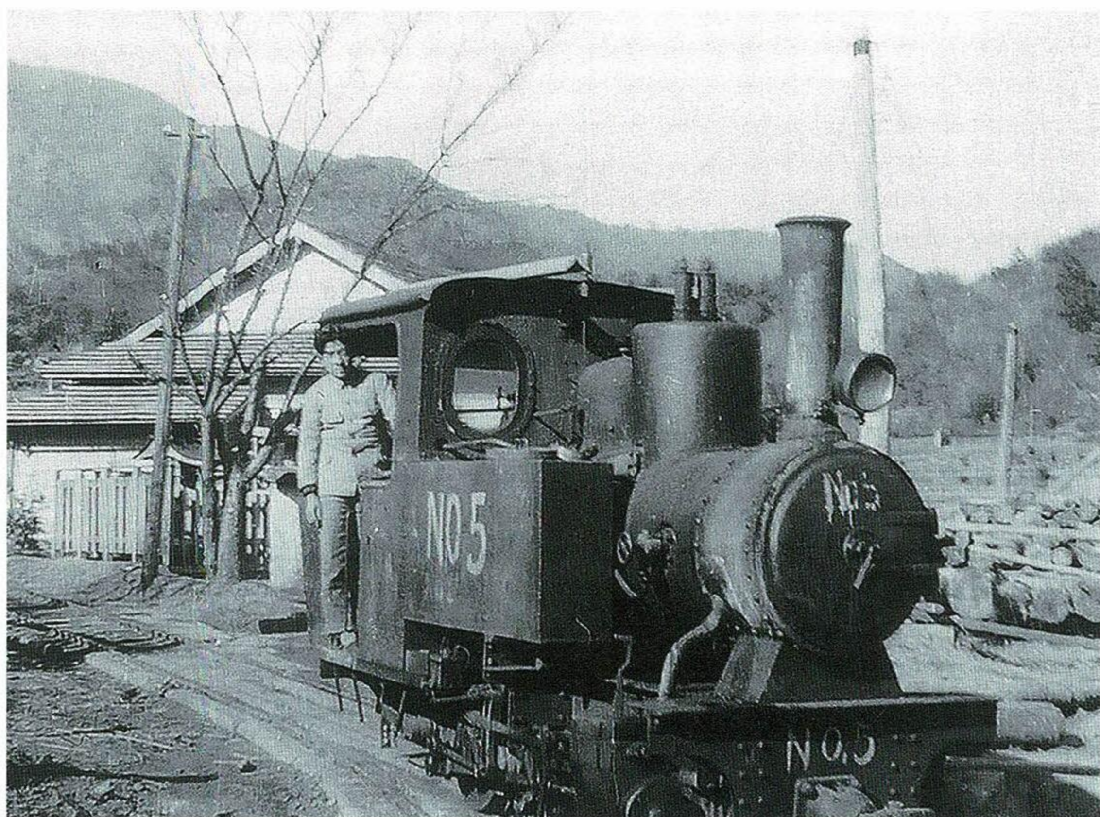
山崎宮林署上野貯木場にて 木材運搬用機関車（喜多寅雄氏 提供）
